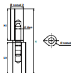
MA... Paumelle MAROC® inox - Bague inox
